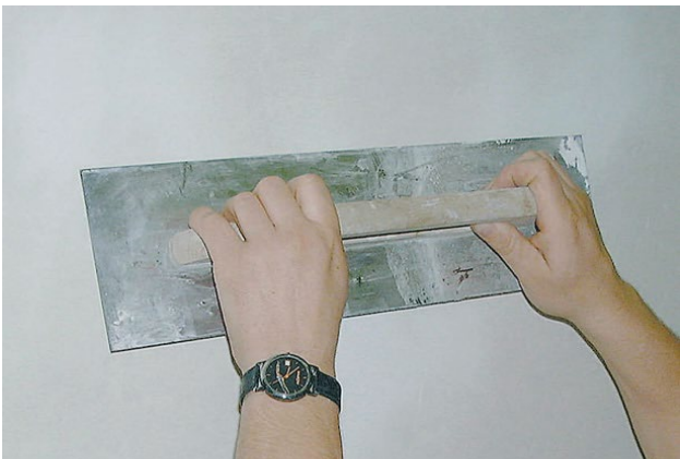
1) Aufbringen des weißen RÖFIX Renoplus®
