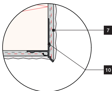
Detail Maßstab 1:2
