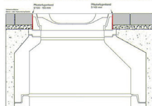
Anwendung: Kontrollschachtabdeckung o.ä. und Pflasterdecken
