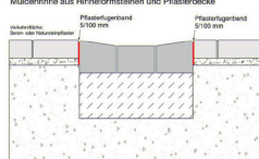
Anwendung: Mülieneinba aus Rinneformsteinen und Pflasterdecke
