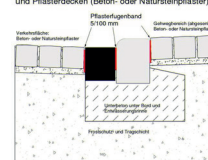
Anwendung: Entwässerungsrinne, abgesenkter Bord (RB) und Pflasterdecken (Biotch- oder Natursteinpflaster)
