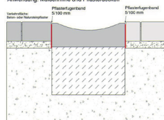
Anwendung: Mülieneinba und Pflasterdecken
