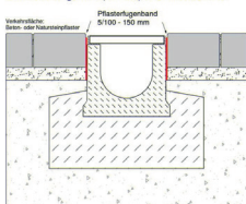
Anwendung: Entwässerungsrinne (NW 200) und Pflasterdecken
