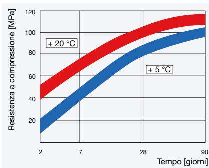
Evoluzione della resistenza a compressione del CLS (con CEM I 42,5 N) in funzione della temperatura del CLS
