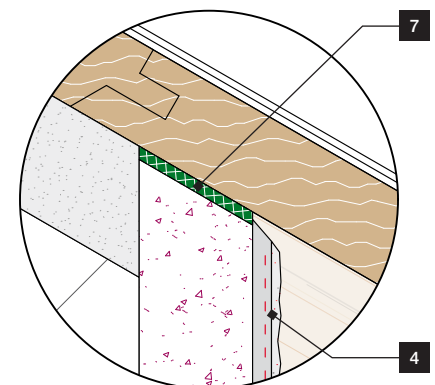
Detail Maßstab 1:2
