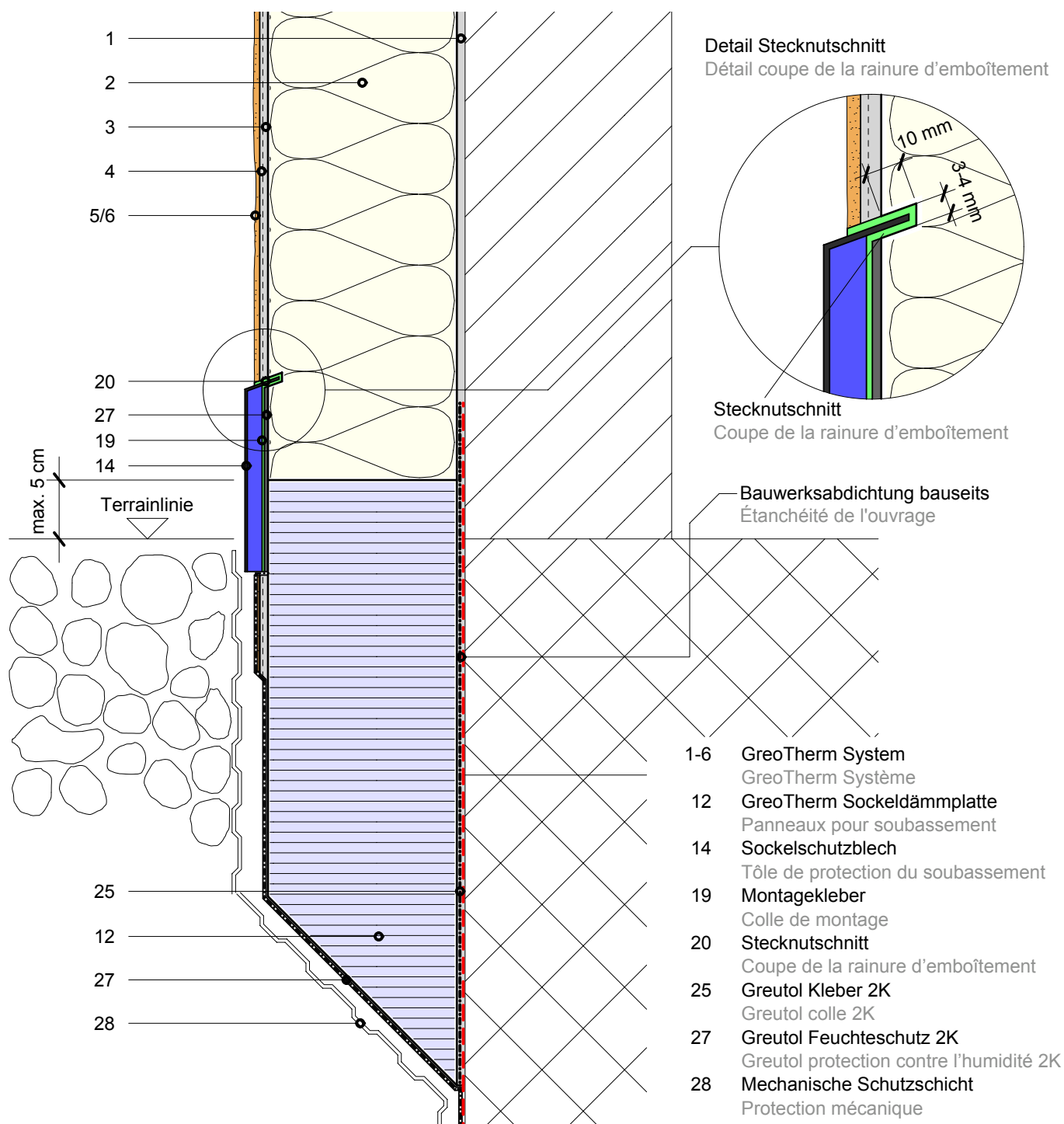
Détail A10
