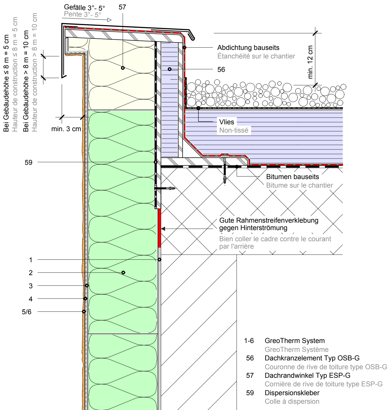
Détail G1
