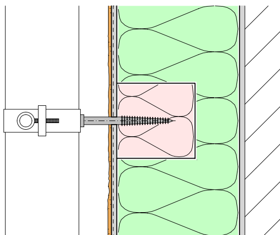
Wärmedämmung Mineralwolle / ZyRillo Montagequader EPS Isolation thermique laine minérale / Carreau de montage ZyRillo EPS
