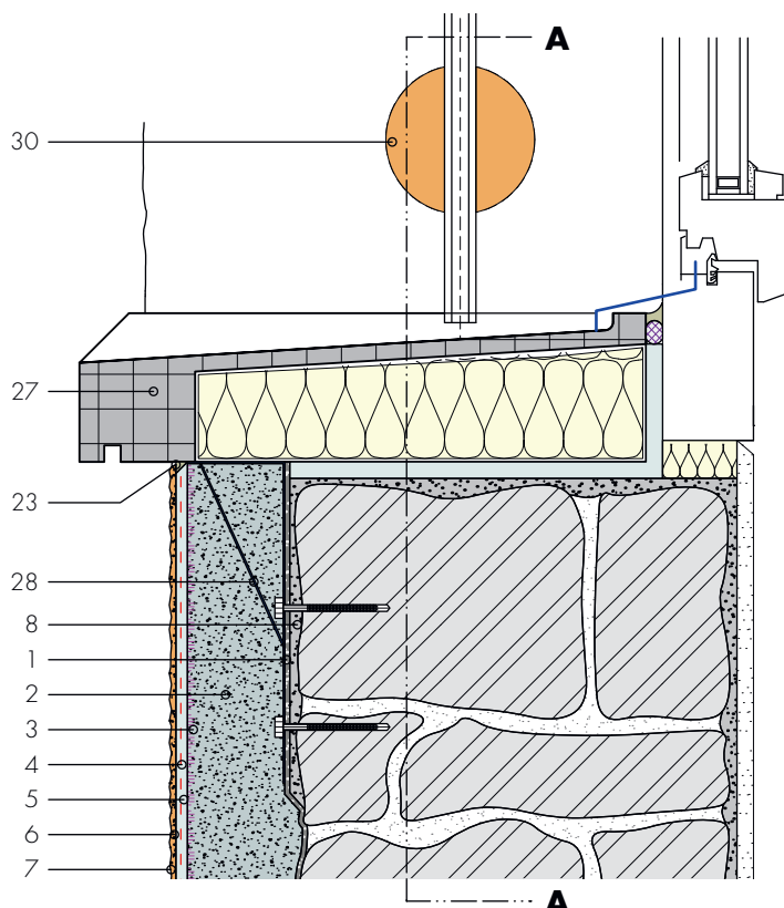
Coupe A-A
