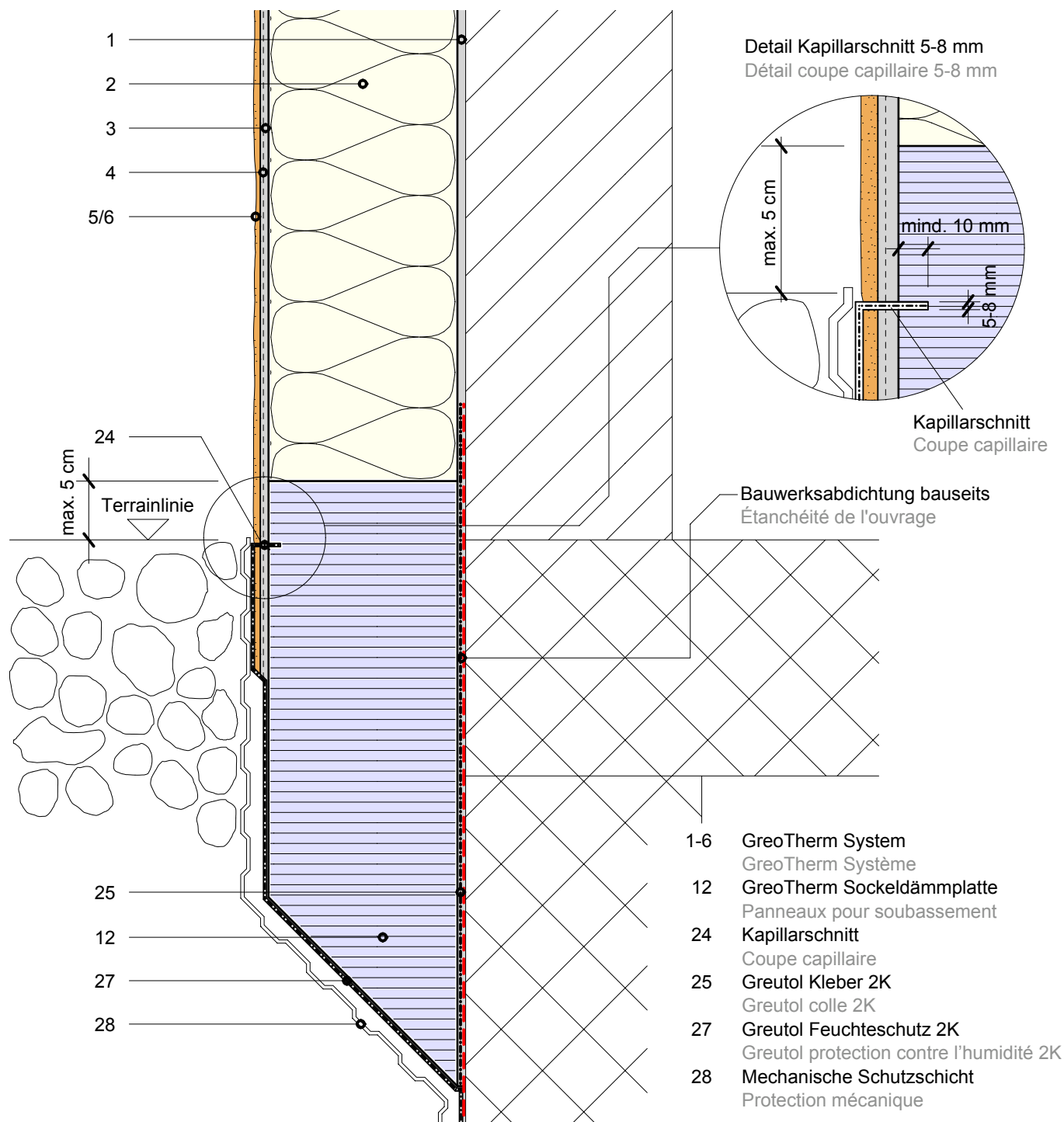
Détail A1
