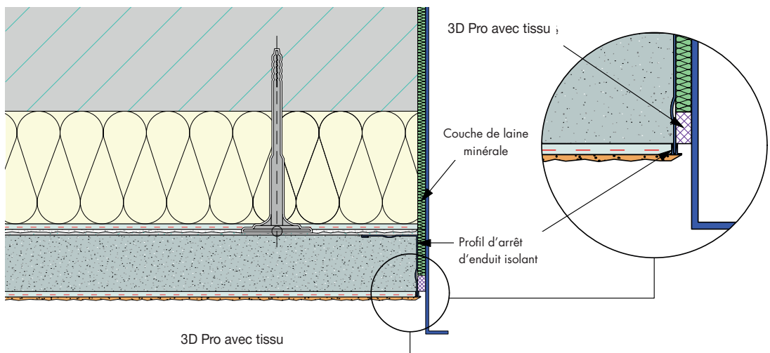
Raccord avec profil d'arrêt (bois)
