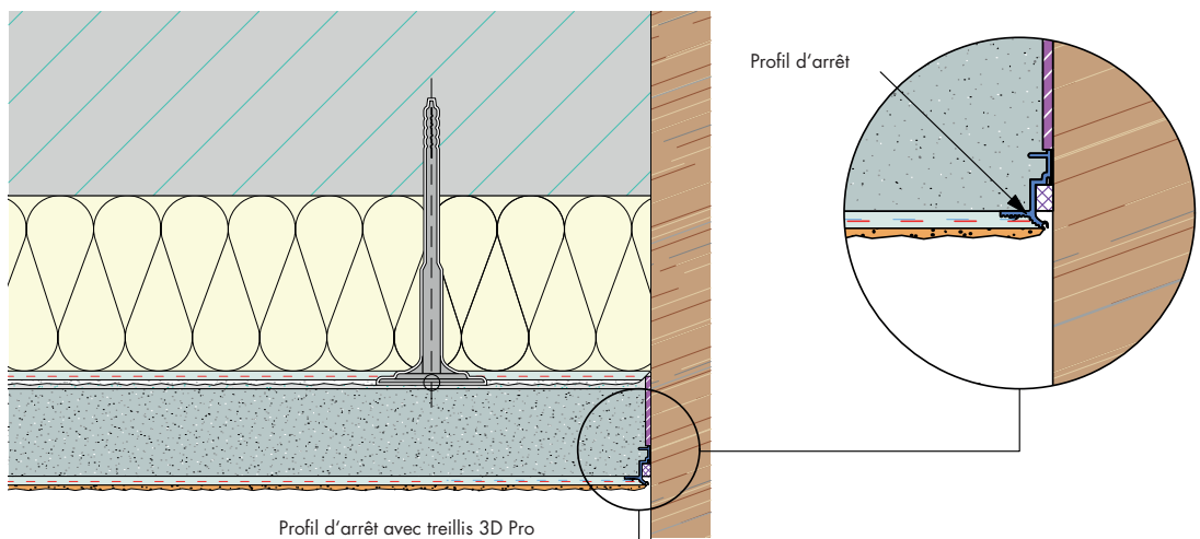
Raccord avec profil d'arrêt (bois)
