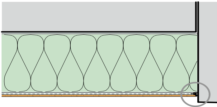
37 Anschlussprofil Ideal Plus
