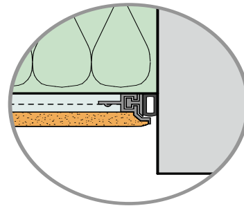
37 Anschlussprofil Ideal Plus
