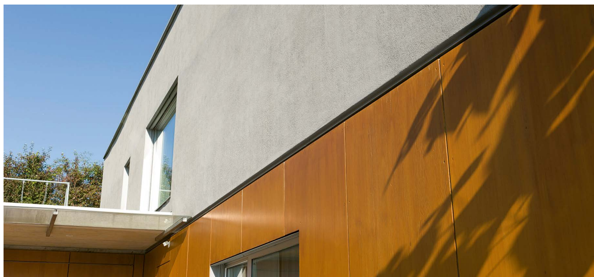
Immeuble d'habitation à Küsnacht, surface : 370 m 2 . Structure du système : isolation avec panneaux lamellaires en laine de pierre, 160 mm; couche de fond Greutol Mortier d'enrobage light 425; enrobage du treillis Greutol Multiplan 407; couche de finition Greutol Enduit de blanchiment light 590 et Enduit de finition résine silicone 361, 5.0 mm.
