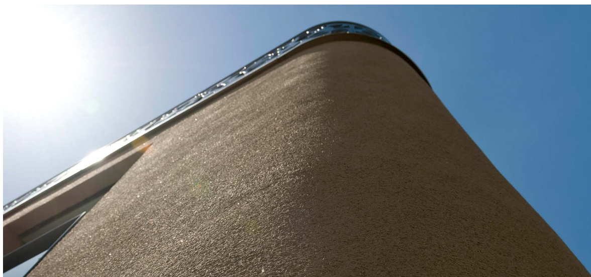
Immeuble d'habitation à Zurich Witikon, surface : 1348m 2 . Structure du système : isolation avec laine de pierre, 240 mm; couche de fond Greutol Mortier d'enrobage light 425; enrobage du treillis Greutol Multiplan 407; couche de finition Greutol Enduit gratté light 585.
