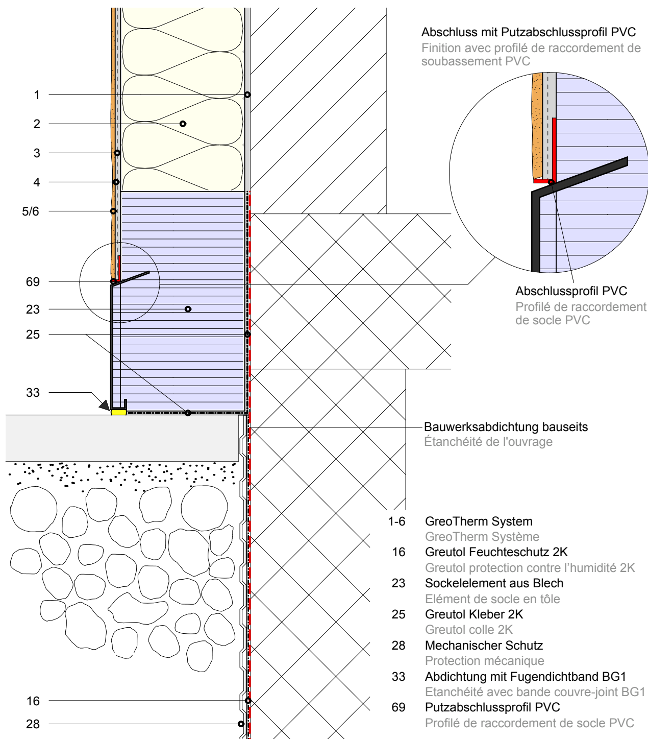
Détail A8
