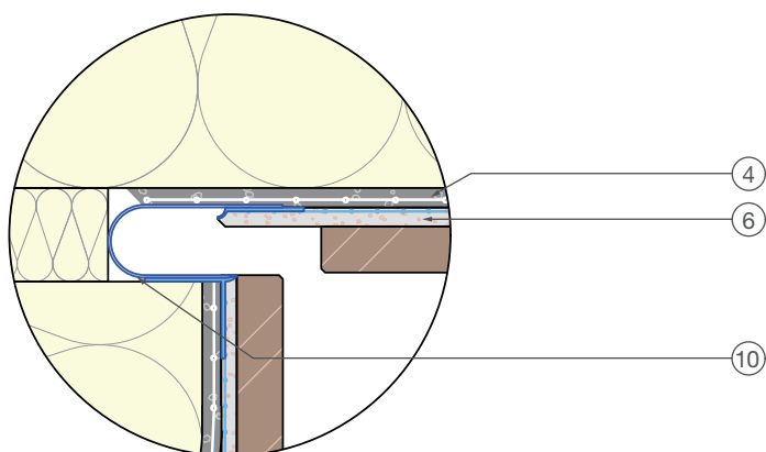
Detail Maßstab 1:2
