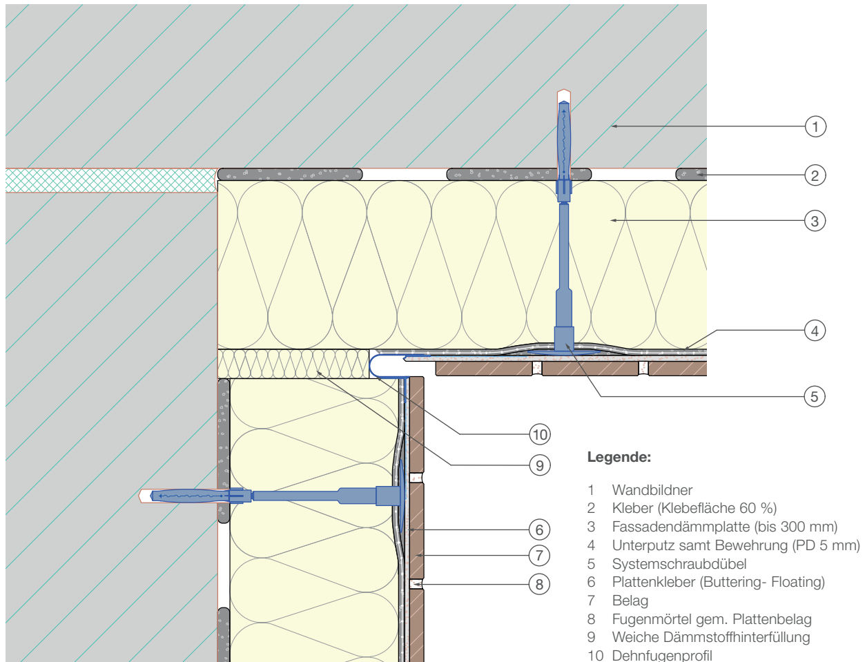
Detail Maßstab 1:2
