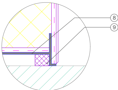
Detail Maßstab 1:2
