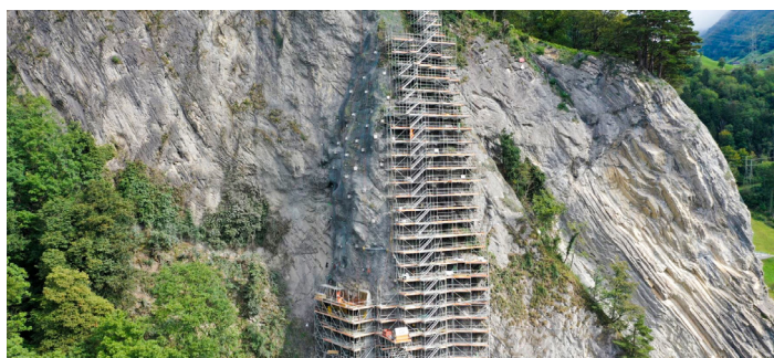
Stabilizarea stâncilor Axenstrasse, Sisikon UR
