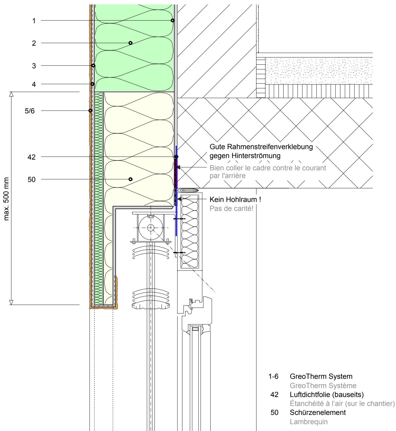
Détail D1
