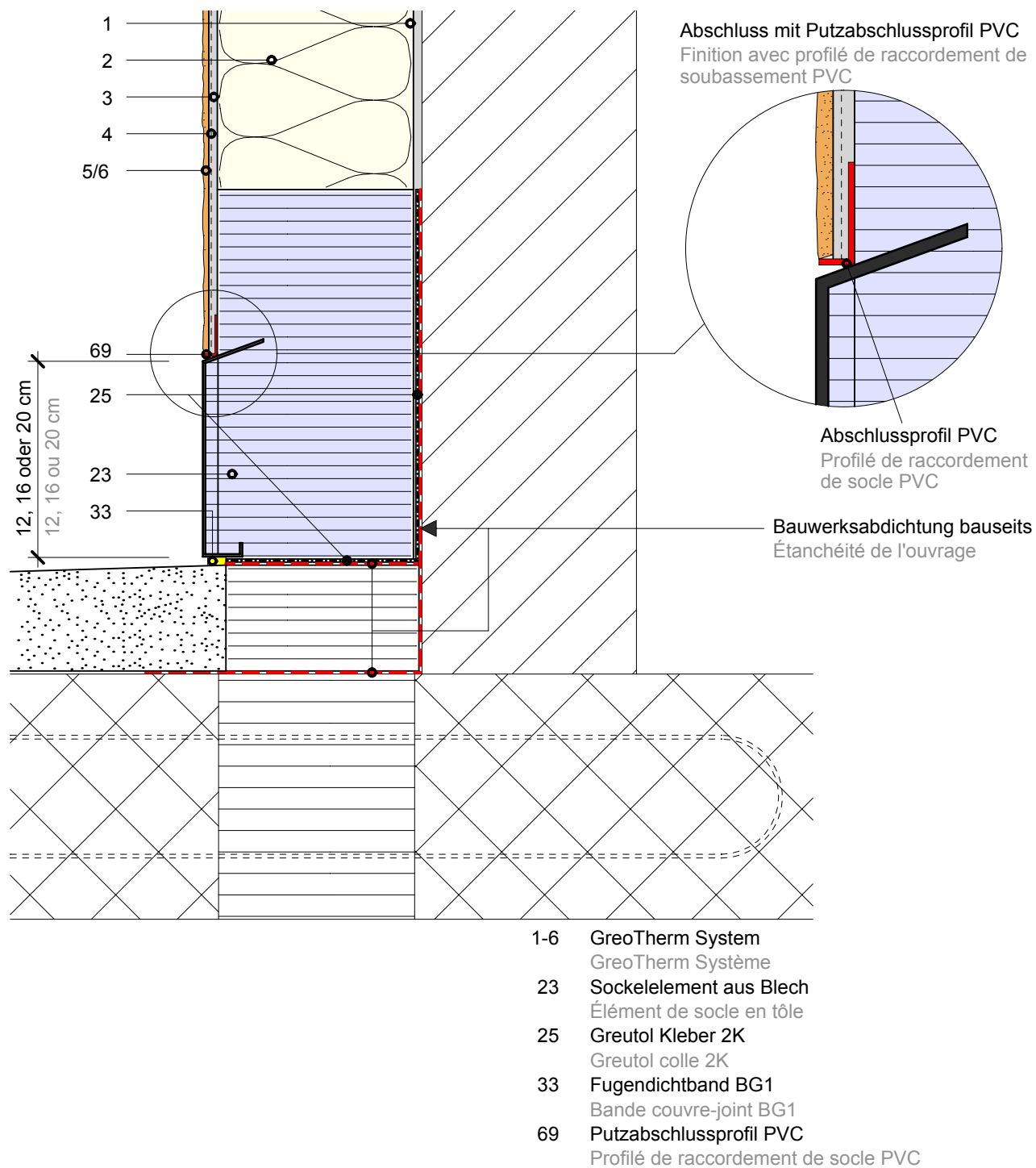
Détail A6
