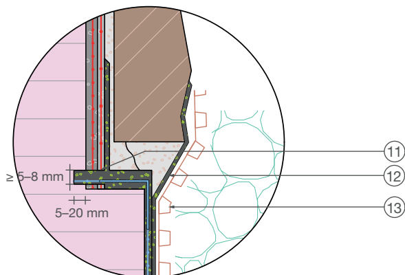
Detail Maßstab 1:2
