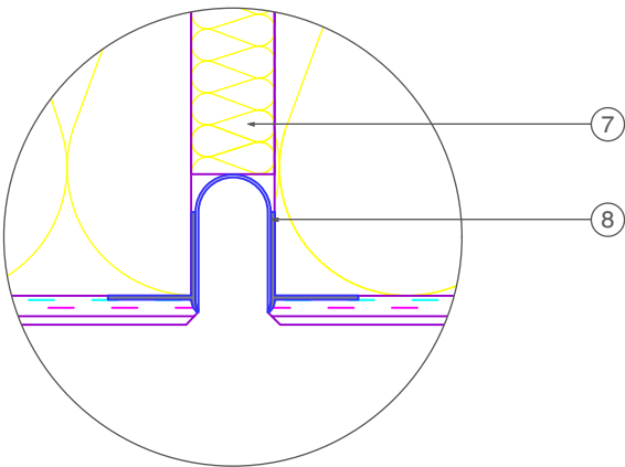
детайл мащаб 1:2
