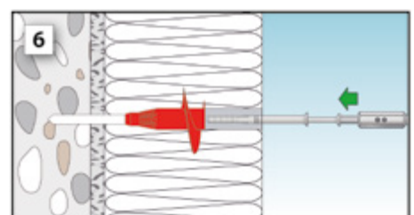
Schraube einstecken
