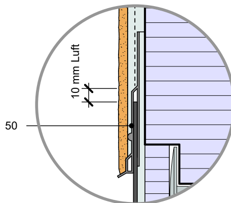
Spenglerblech ohne Umschlag
