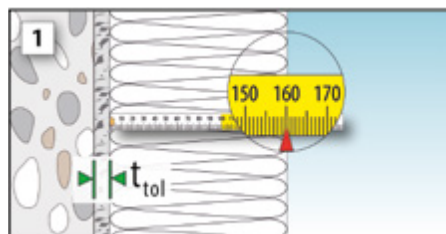
Dämmdicke messen
