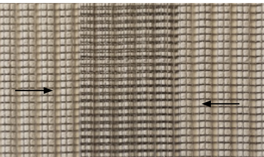
Netzüberlappung min. 10 cm
