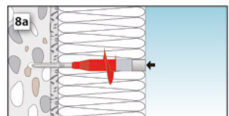
Loch verschliessen
