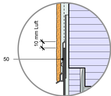
Spenglerblech ohne Umschlag
