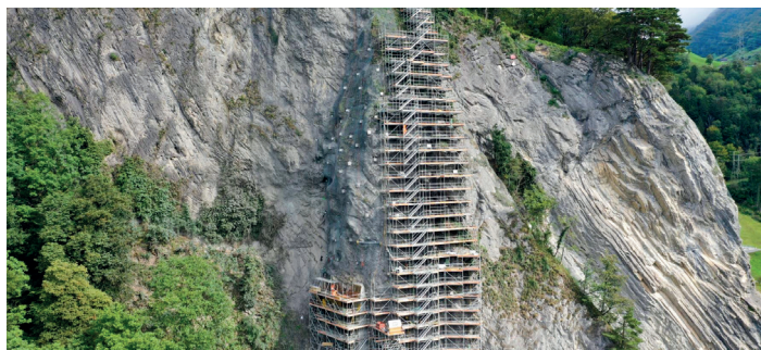
Sécurisation de la route « Axenstrasse », Sisikon UR
