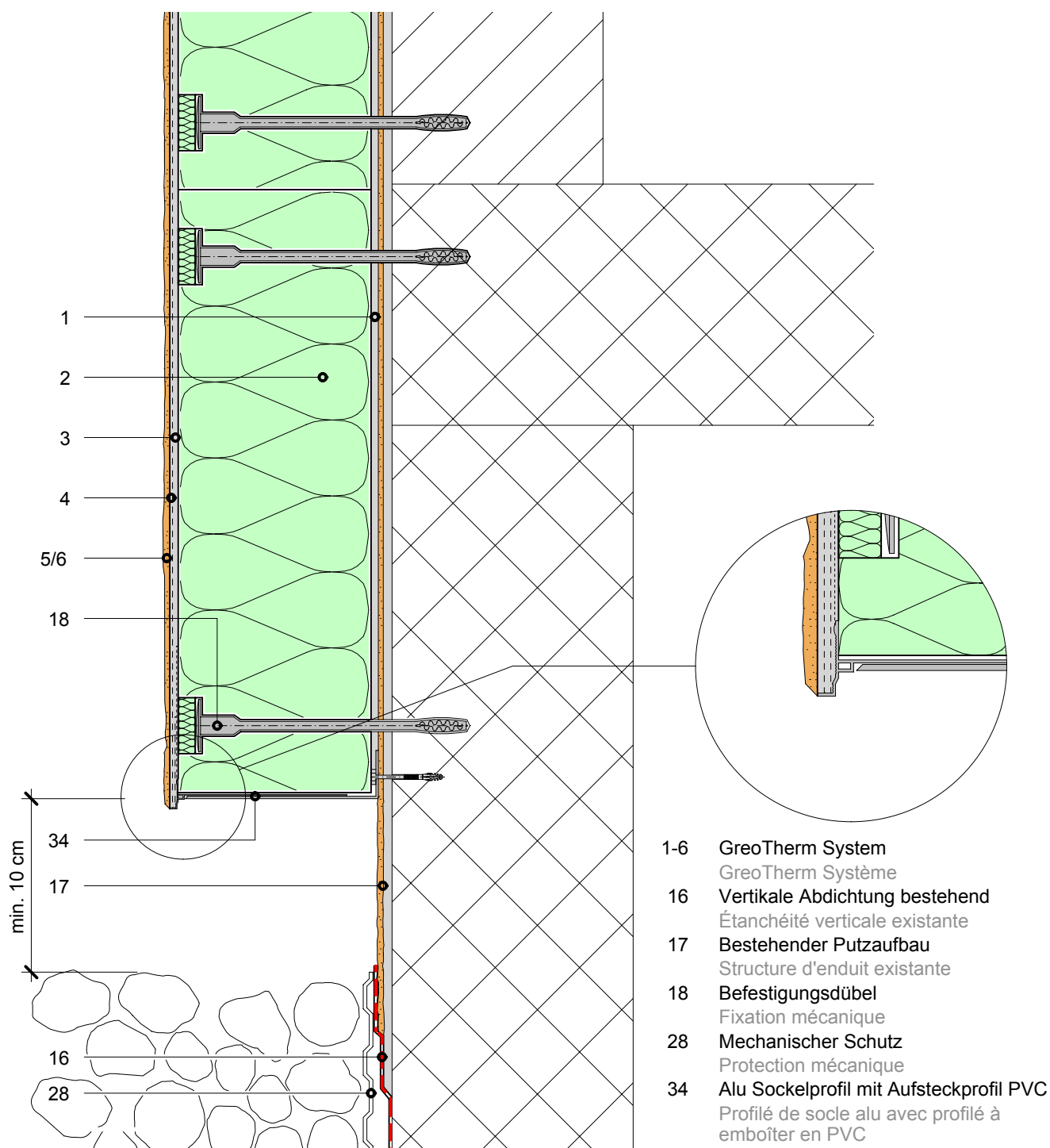
Détail A11
