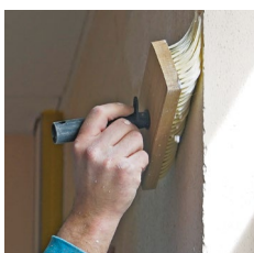
4 Auftragen des Verfestigers
