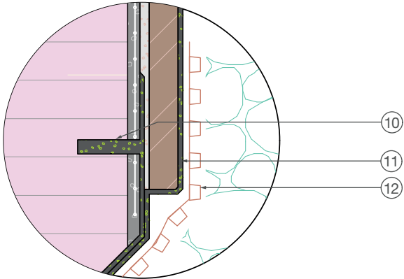
Детайл Мащаб 1:2
