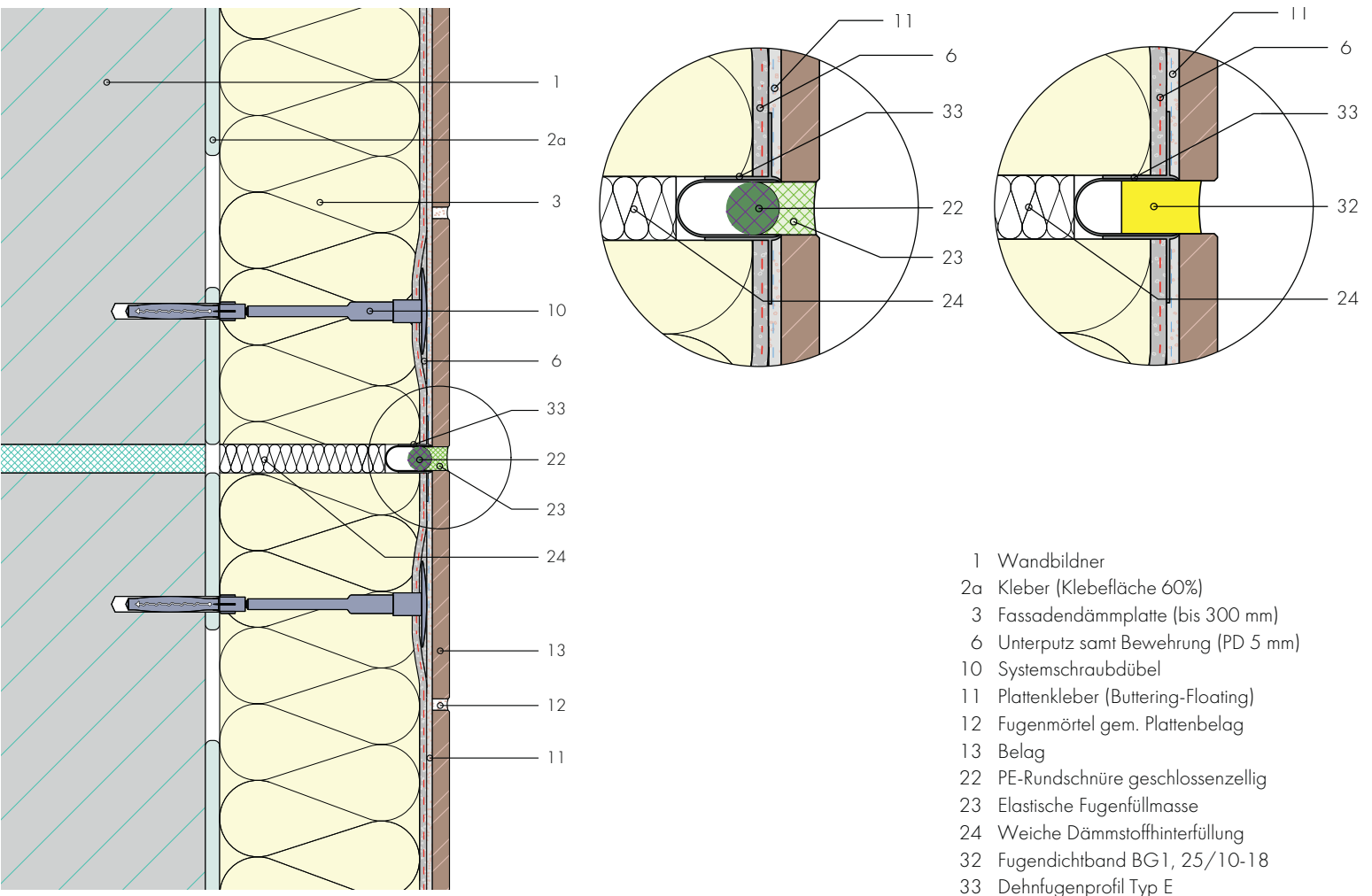
S.9.5 Gebäudetrennfuge mit Fugendichtband/BG1
