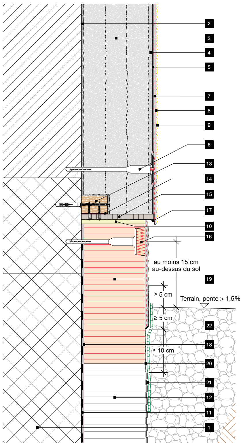
Détail A1
