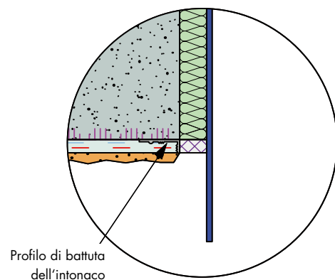
Raccordo per telaio metallico con nastro per giunti BG1
