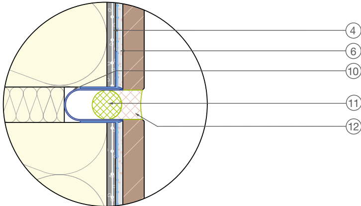
Detalj Omjer 1:2
