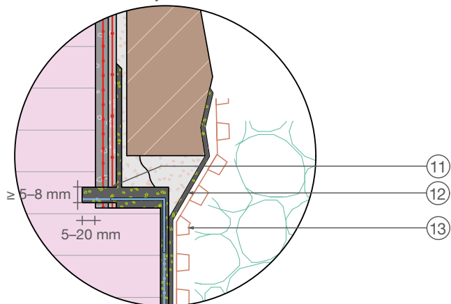
Detalj Omjer 1:2
