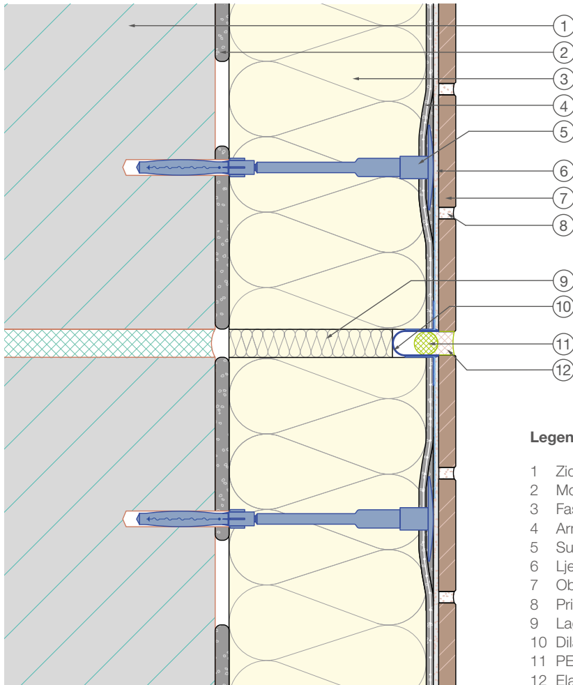
Detalj Omjer 1:2
