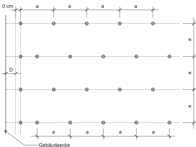
S.10.1 Dübelanordnung bei oberflächenbündiger Montage durch das Gewebe.
