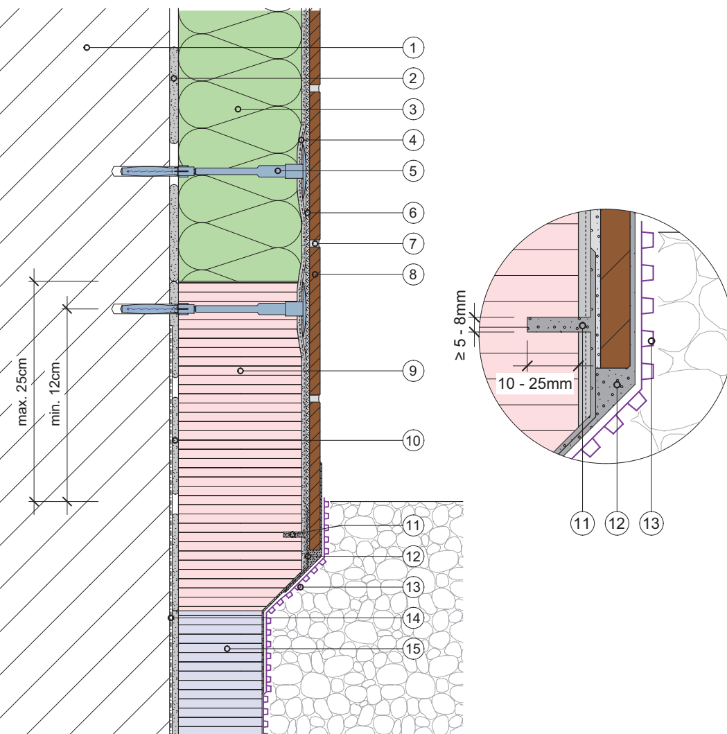
S.1.1 Sockel mit Kapillarschnitt
