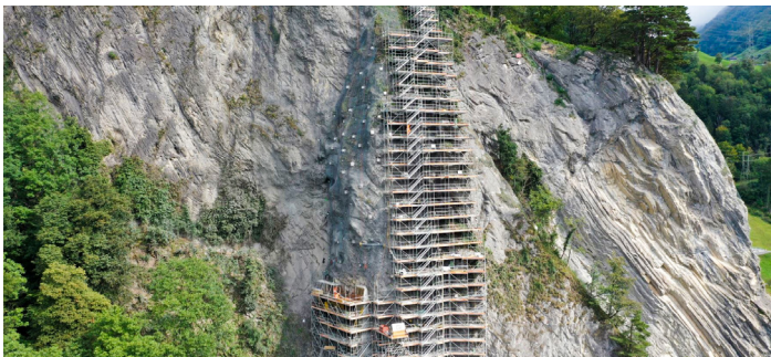
Uolų stabilizavimas Axenstrasse, Sisikon UR
