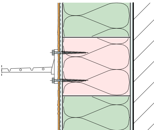
64 Montagequader Quadroline® EPS 150 x 100 mm (verklebt mit Systemkleber auf den Untergrund)
