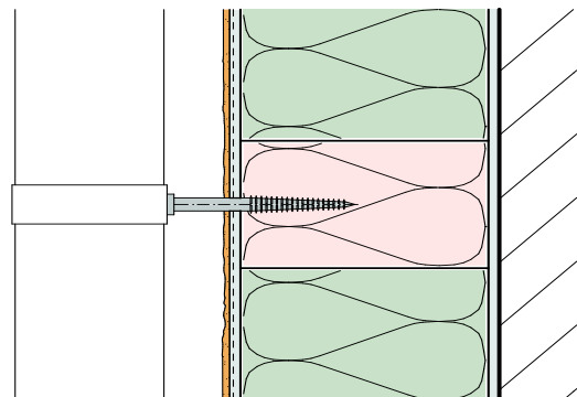
65 Montagequader Quadroline® EPS 100 x 100 mm (verklebt mit Systemkleber auf den Untergrund)
