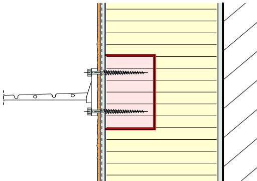
62 Montagezylinder ZyRillo® Ø 125 mm
