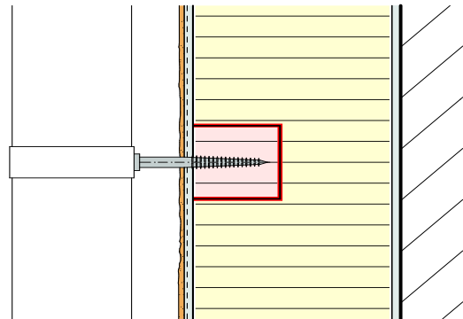
63 Montagezylinder ZyRillo® Ø 70 mm
