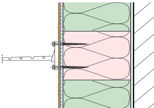
64 Montagequader Quadroline® EPS 150 x 100 mm (verklebt mit Systemkleber auf den Untergrund)
