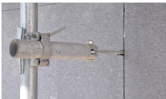
Ancrage de l'échafaudage
