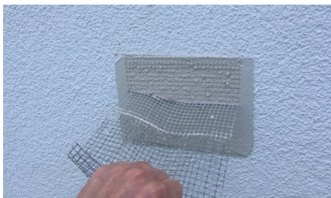
Préparation pour l'essai d'arrachage
