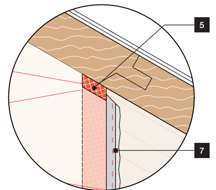
Detail Maßstab 1:2
