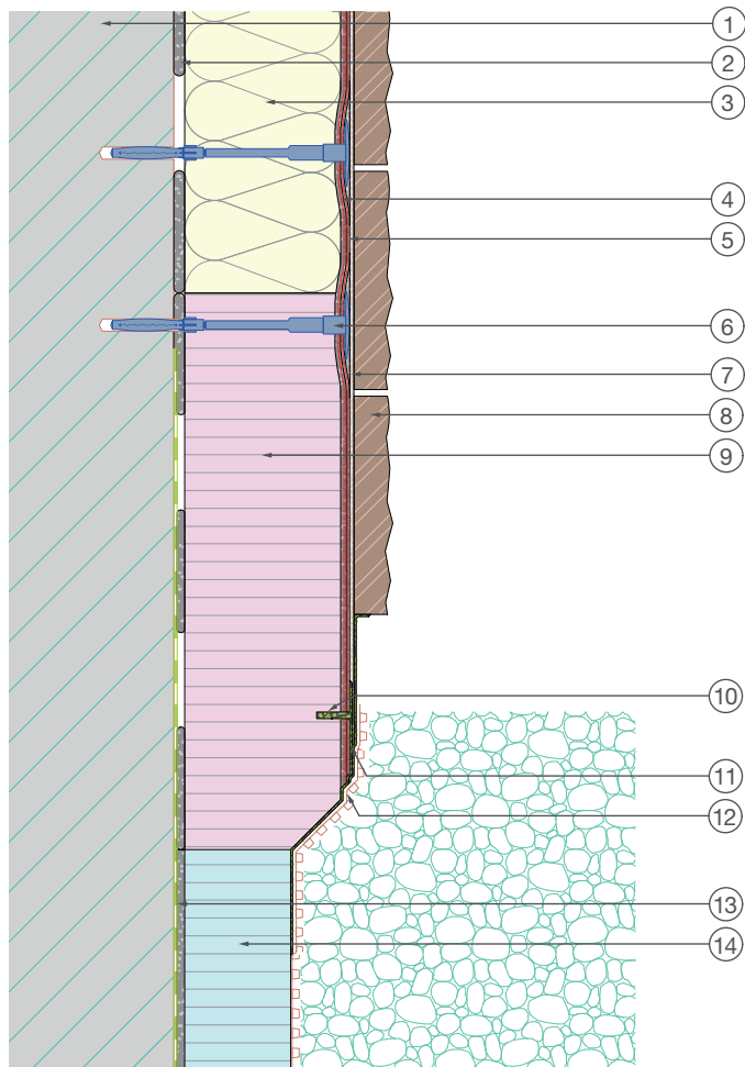
Detail Maßstab 1:2
