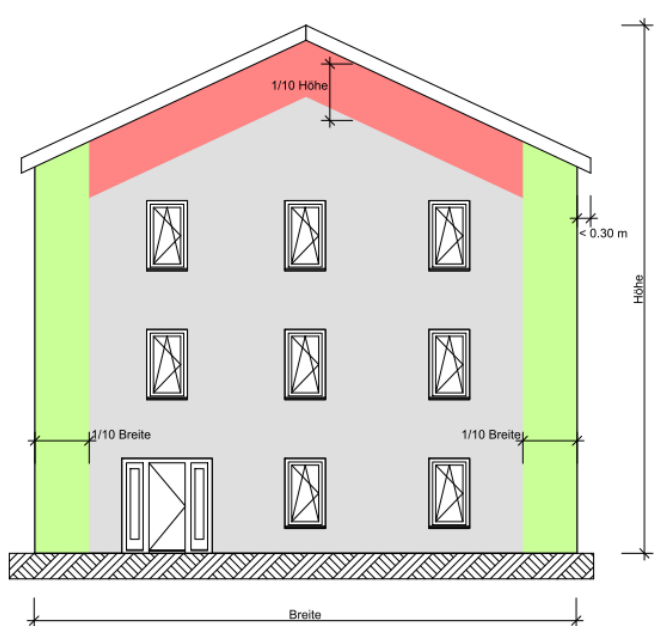
Dachüberstand < 0.3\text{ m} (Traufe und/oder Giebel)
