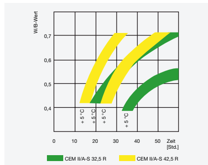
Erforderliche Zeit zum Erreichen der Gefrierbeständigkeit des Betons. (Betondruckfestigkeit > 5 N/mm 2 in Abhängigkeit vom w/z-Wert bei verschiedenen Betontemperaturen und Zementarten)
